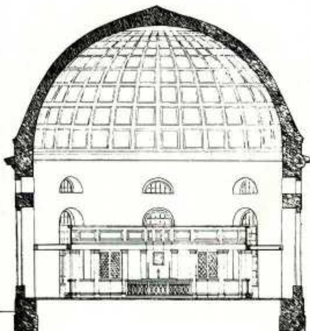
Hohenzieritz, Schnitt
